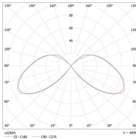
KANLUX S.A. (kat 36557) SELTO EL 23 B + IQ-LED / LDC (Polar)
